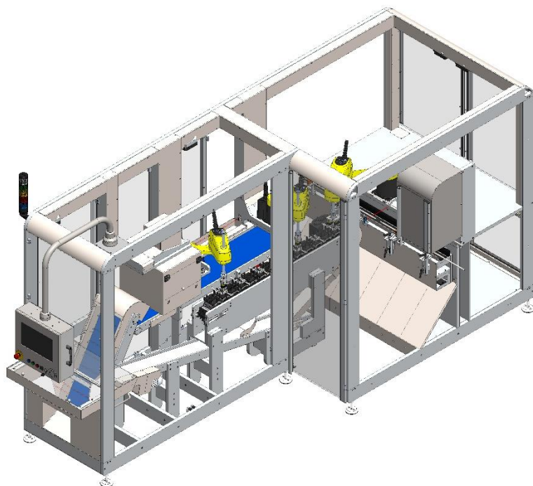
Exemple d'un module d'alimentation seringues en vrac, avec dépose au pas et en quinconce + insertion des seringues dans l'étui et contrôle présence et intégrité des seringues
