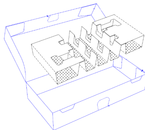
Exemple d'étui traité par la machine : étui coffret avec chevalet pour simple et double seringues
